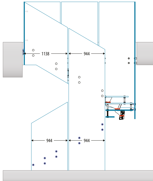
COUPE A-A'
