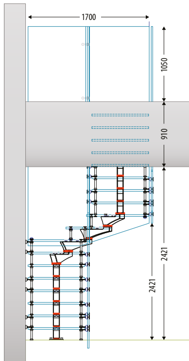
VUE FRONTALE
