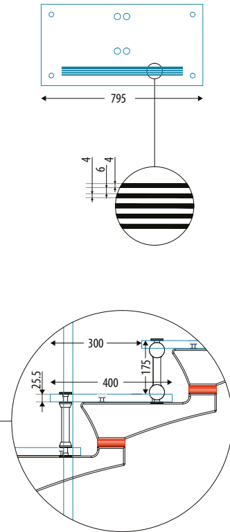
SÉRIGRAPHIE MARCHES
